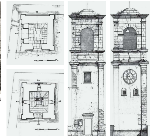
Σχέδια αποτύπωσης Κ. Παραθουρά 1994 (Πηγή: Στανέλλος Λ., 2015)
