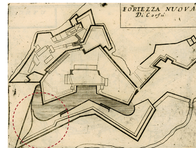
Επισημαίνεται η θέση του ημιπρομαχώνα σε κάτοψη του Νέου Φρουρίου της Κέρκυρας. Εντοπίζονται διαφορές στο περίγραμμα του Σκάρπωνα, οι οποίες ενδεχομένως οφείλονται στην ανακατασκευή του οχυρού το 1728. CORONELLI, Βενετία, 1688. (Πηγή: Ίδρυμα Αικ. Λασκαρίδη)
