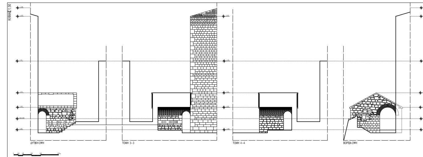
Όψεις και τομές της υφιστάμενης κατάστασης της νότιας καπονιέρας της τάφρου (αποτύπωση 2013) (Πηγή: Στανέλλος Λ., 2015)
